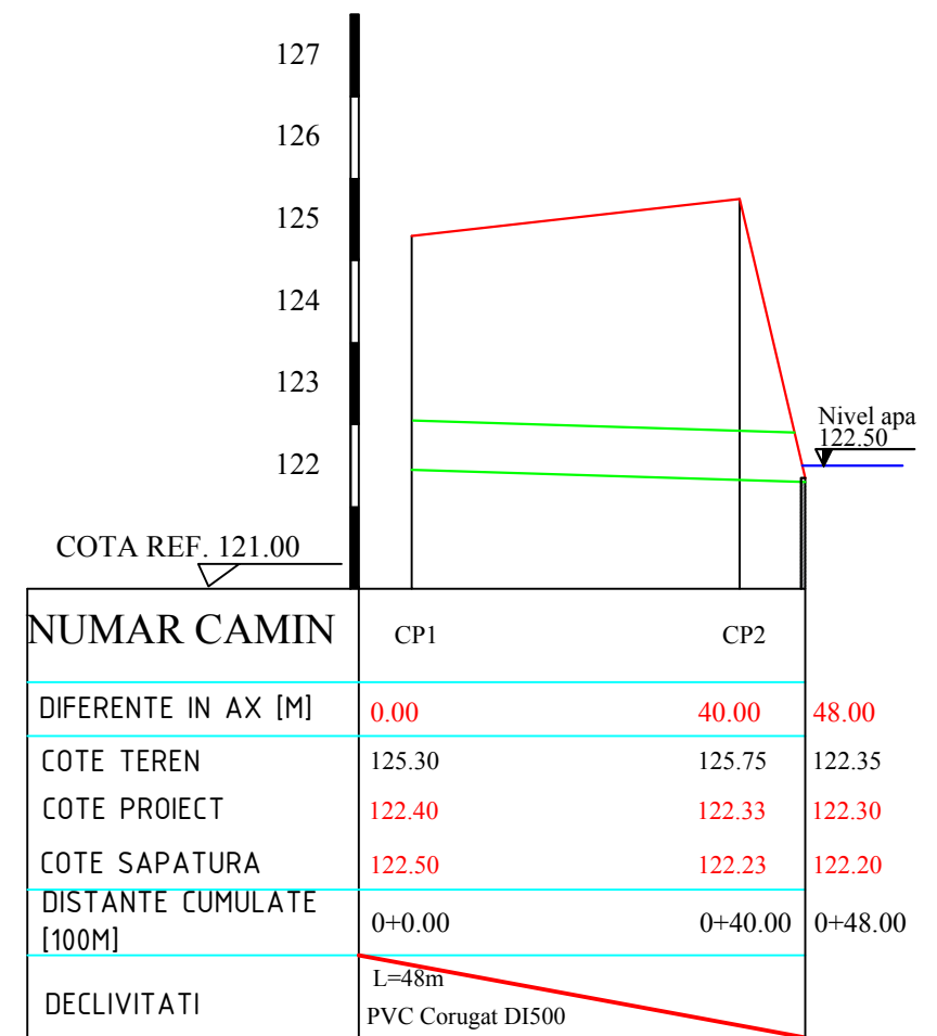
PROFIL LONGITUDINAL : CANALIZARE PLUVIALA SCARA 1:100 / 1: 1000
