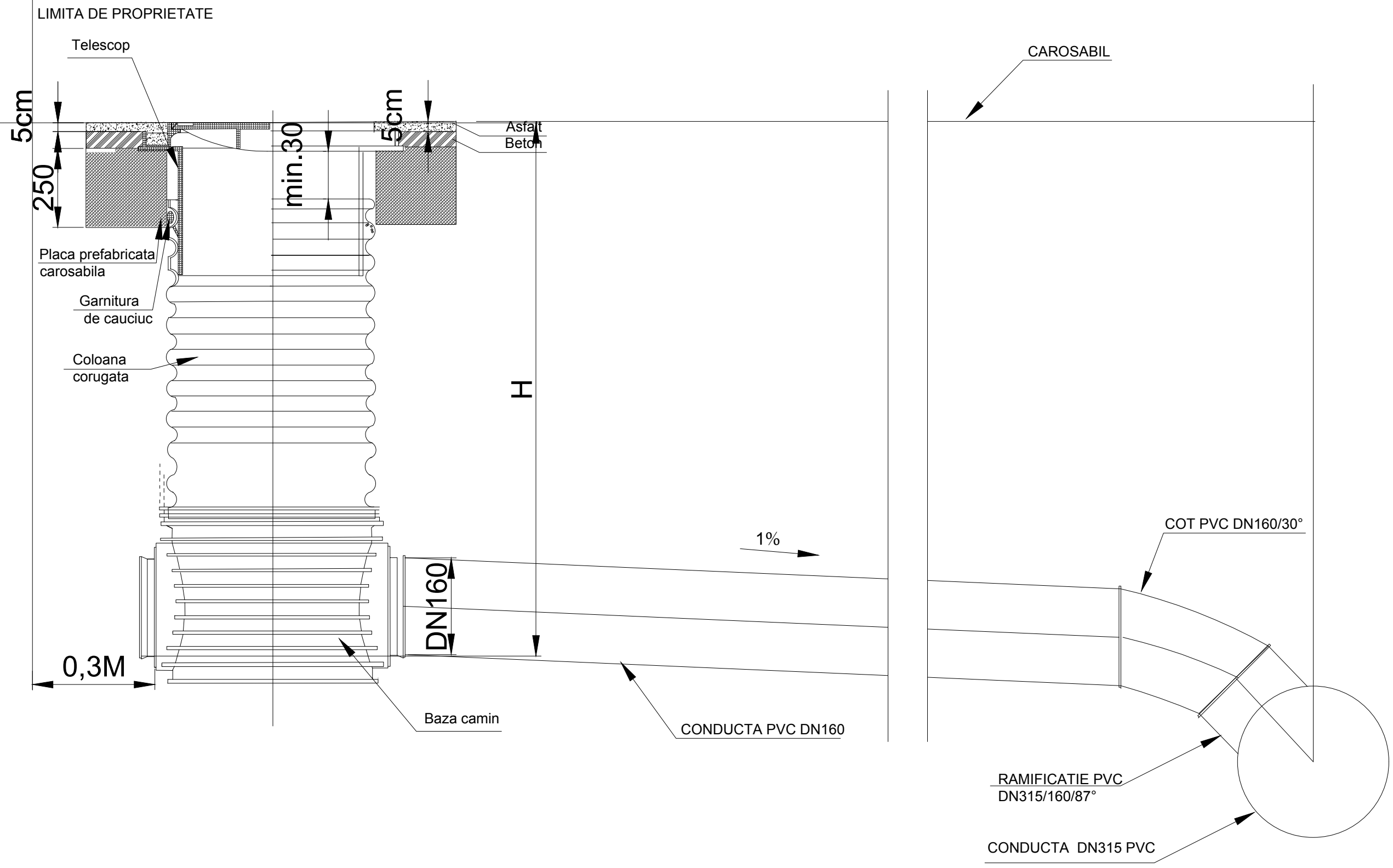
CAMIN DE RACORD DN300 H DE LA 1M LA 1,5M
